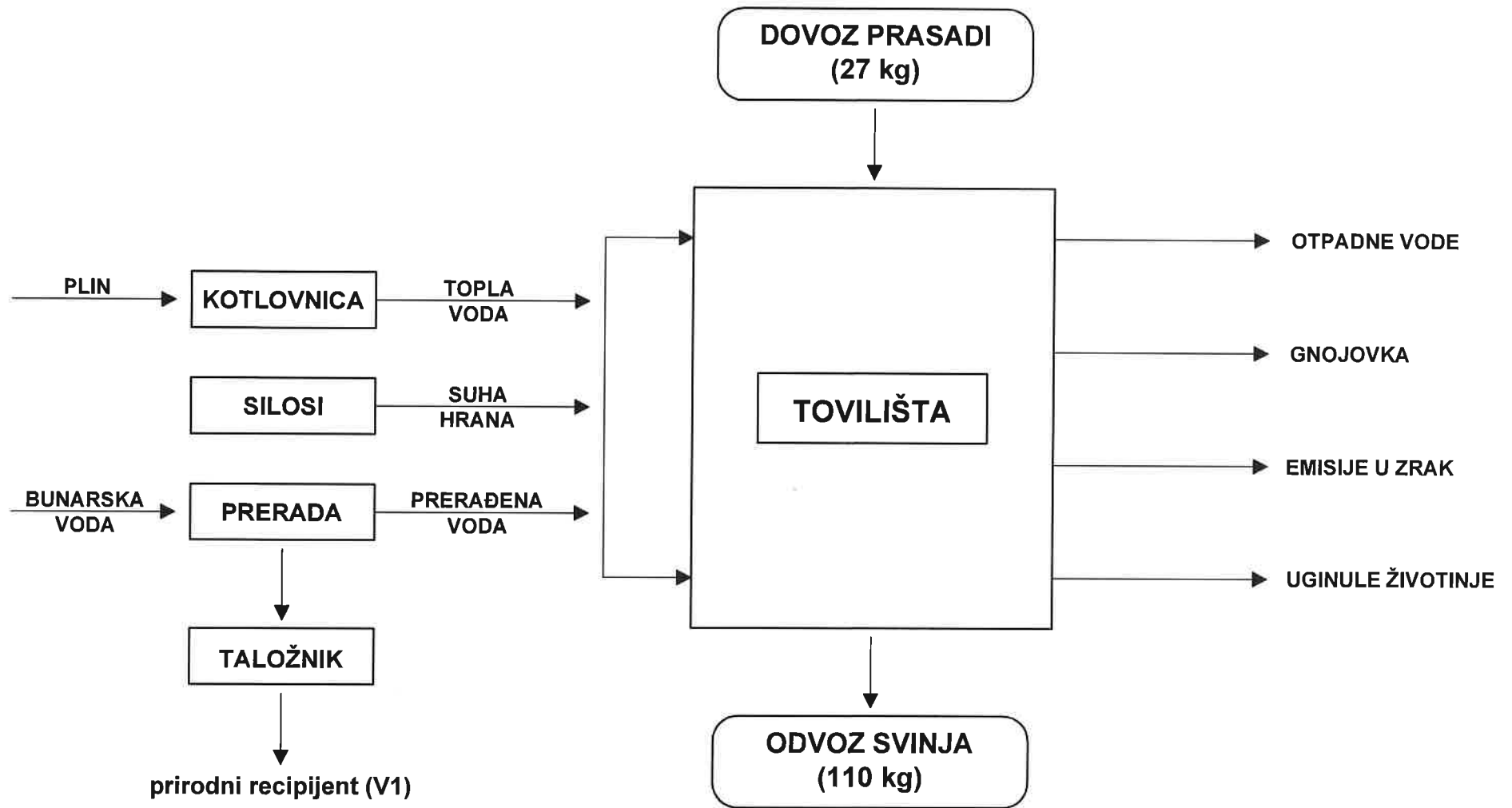
Prilog 2. Blok dijagram tehnološkog procesa na Farmi Darda 1
